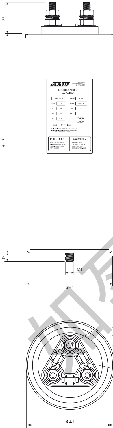
Condensatore ø 120 mm Capacitor ø 120 mm
