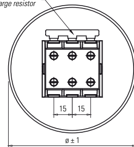
Resistenza di scarica Discharge resistor
